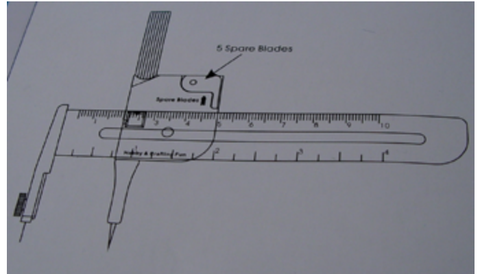
510 091 Kreisschneider mit Ersatzmesser VE 3
